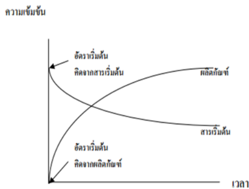
รูปที่ 8.4 การเปลี่ยนแปลงความเข้มข้นของสารที่เข้าทำปฏิกิริยา [8]
