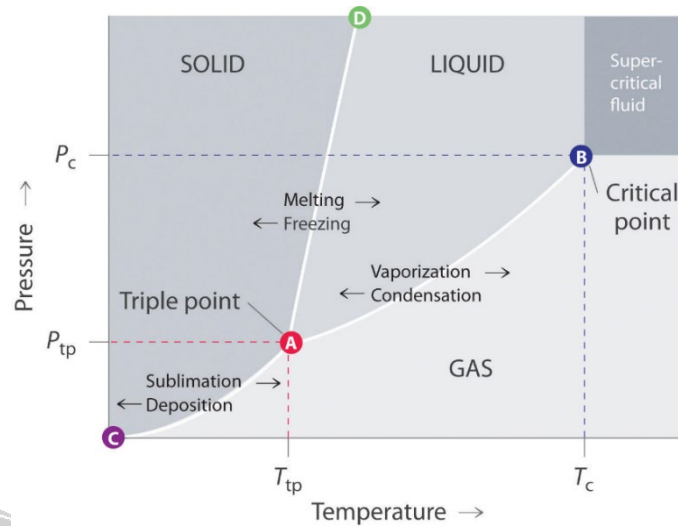
รูปที่ 5.1 แผนผังวัฏภาค (Phase diagram) [7]
